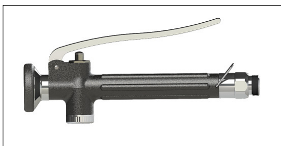
ES(1.4305)-Handbrause mit Metallkopf, G 1/2'' AG Durchflußmenge 9 ~ 15 Ltr/min; 2-4Bar
